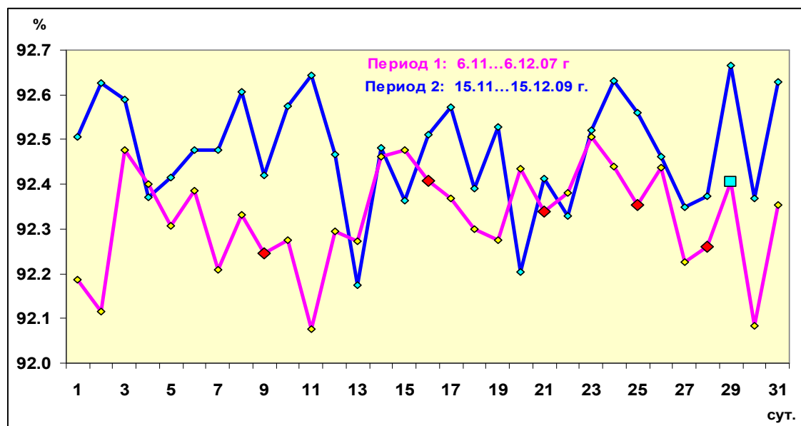
Рис.7. Сопоставление динамики относительной \gamma -активности образца №25 (относительно контрольного образца) в 2-х периодах (фрагменты характеристик). Даты воздействия отмечены красными ромбами. Дата реверса Потока ИП отмечена голубым квадратом.
