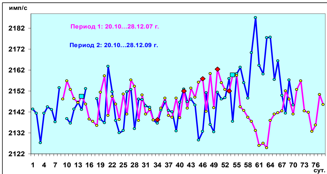
Рис.2. Сопоставление динамики \beta -активности образца №25 в 2-х периодах (приведенные значения):
