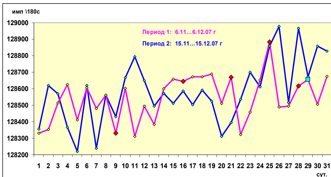
Рис.6. Сопоставление динамики \gamma -активности образца №25 в 2-х периодах (фрагменты характеристик). Приведенные значения. (Даты воздействия отмечены красными ромбами. Дата реверса Потока ИП отмечена голубым квадратом).
