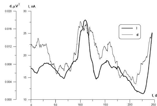
Рисунок 5: Синхронные вариации сигналов фотокатодного детектора I (толстая линия) и детектора подвижности ионов d (тонкая линия): t — время в сутках. Реализация 17.01.1997 – 19.09.1997.
