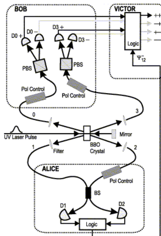
Рисунок 4: Схема эксперимента. Пары запутанных фотонов генерировались при прохождении импульса ультрафиолетового лазера через кристалл ВаВ2О4. После спектральной фильтрации фотоны поступали в одномодовое оптоволокно и направлялись Бобу и Алисе.
