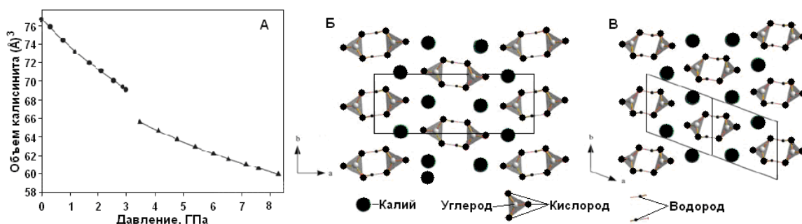
Рис. 2. Изменение удельного объема ( \Delta V/V = 4\% ) в калисините при давлении 3.2 ГПа –А, изменение пространственной структуры калисинита - Б, В. [6].
