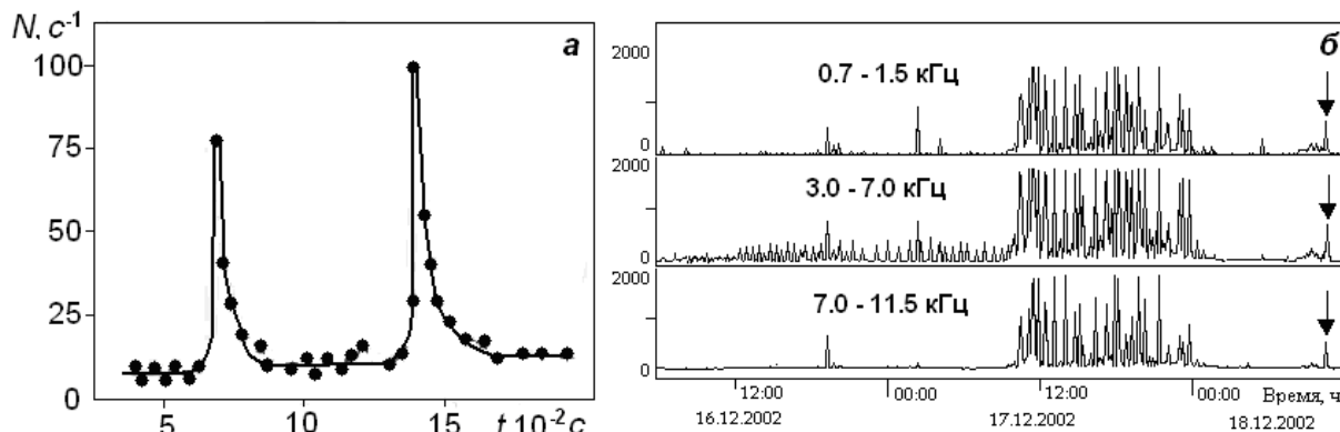
Рис. 1. а) Скорость образования трещин в диабазе при действии на образец постоянного одноосного сжимающего напряжения [2]. б) Акустические сигналы, зарегистрированные перед землетрясением 18.12.2002 ( K = 12.1 ) на Камчатке (ИКИР ДВО РАН). Время события отмечено стрелкой [5].
