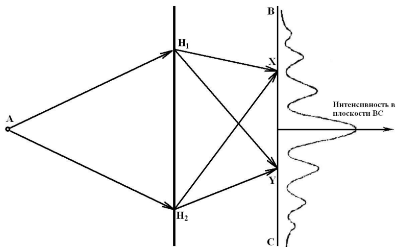
Рис.2. Интерференционная картина с волновой точки зрения
