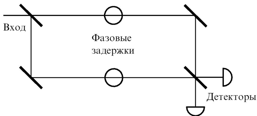
Рис.3. Схема интерферометра Маха-Цандера.
