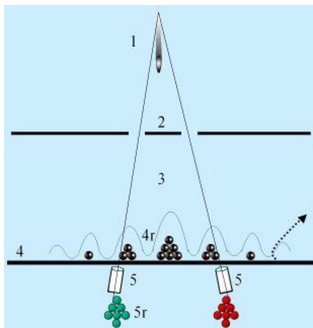
Рис.5. Базовый вариант отложенного выбора
