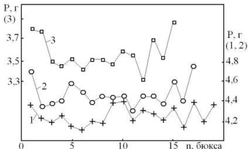
Рис.2. Вес испарившейся воды (1, 3) и спирта (2) из бюксов ( \varnothing = 2 см, h = 3 см), линии которых ориентированы с востока на запад. 1 – водопроводная вода выстоянная сутки, время испарения t = 10 суток; 2 – этанол, t = 4 суток; 3 – вода + сахар (40%), t = 7 суток.
