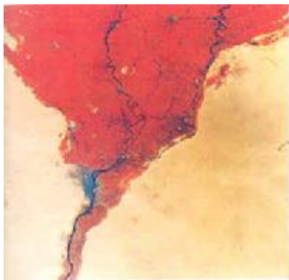
Рис. 3. Космическая фотография дельты Нила в инфракрасном диапазоне. Красным цветом выделяются области, покрытые растительностью, включая возделываемые поля [12].
