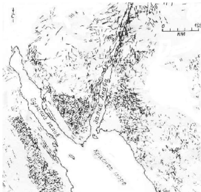
Рис. 4. Схема разрывных структур для районов заливов Суэцкого и Акаба [13].
