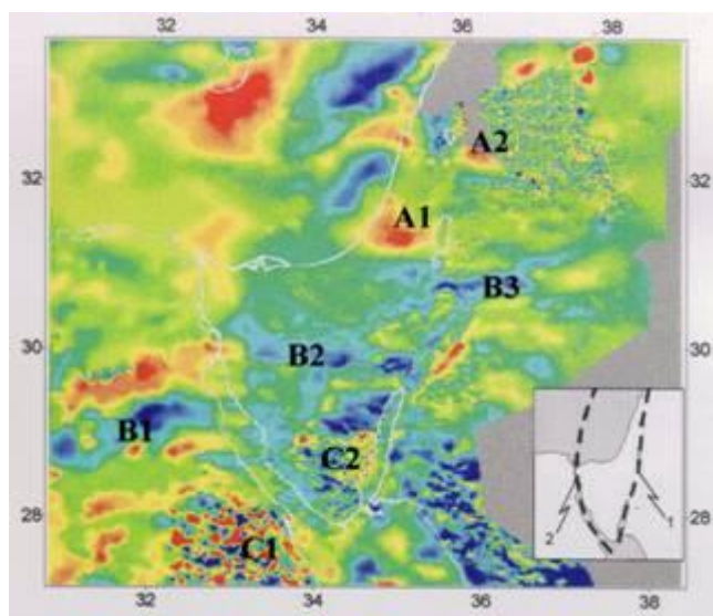
Рис. 2. Карта современного магнитного поля региона Средиземного и Красного морей; на врезке – тектонические линии рифтовых зон (1 - Мертвого моря, 2 – Суэцкого залива) [11]. Магнитные аномалии, связанные с магматическими телами разного состава, A1 и A2 (красных - положительных), B2 и B3 (синих - отрицательных) вдоль Мертвого моря, а также B1 и B2 (синих - отрицательных), C1 и C2 (переменных) связанных с вулканическими базальтами, вдоль Суэцкого залива.
