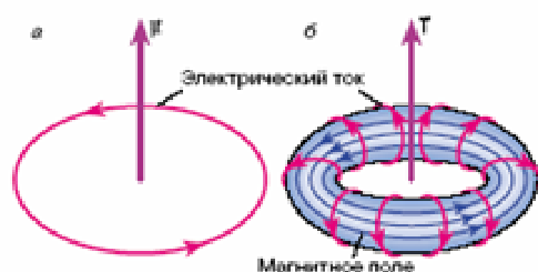
Рис.2. Схемы конфигураций электрического тока и магнитного поля в магнитном ( \mu ) и анапольном моменте (Т).
