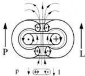
Рис.5. Схема левоспирального нейтрино ( S = \hbar/2 ). Внутренняя v/g -орбиталь является двигателем нейтрино, работающим по принципу водометного двигателя. v/g -Вихрь эфира с импульсом p (дорожка Кармана) движется по инерции. Стрелками показаны циркуляции непрерывных потоков эфира.
